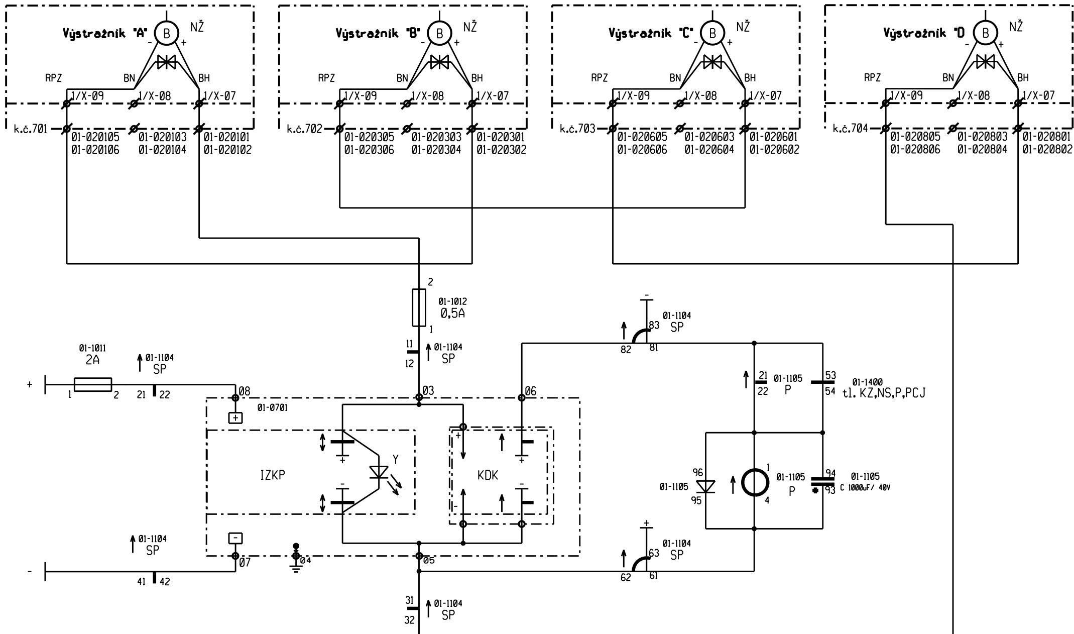
Zapojení PZZ-K VÝKRES ČÍSLO : Zapojení pozitivní signalizace 8202.
